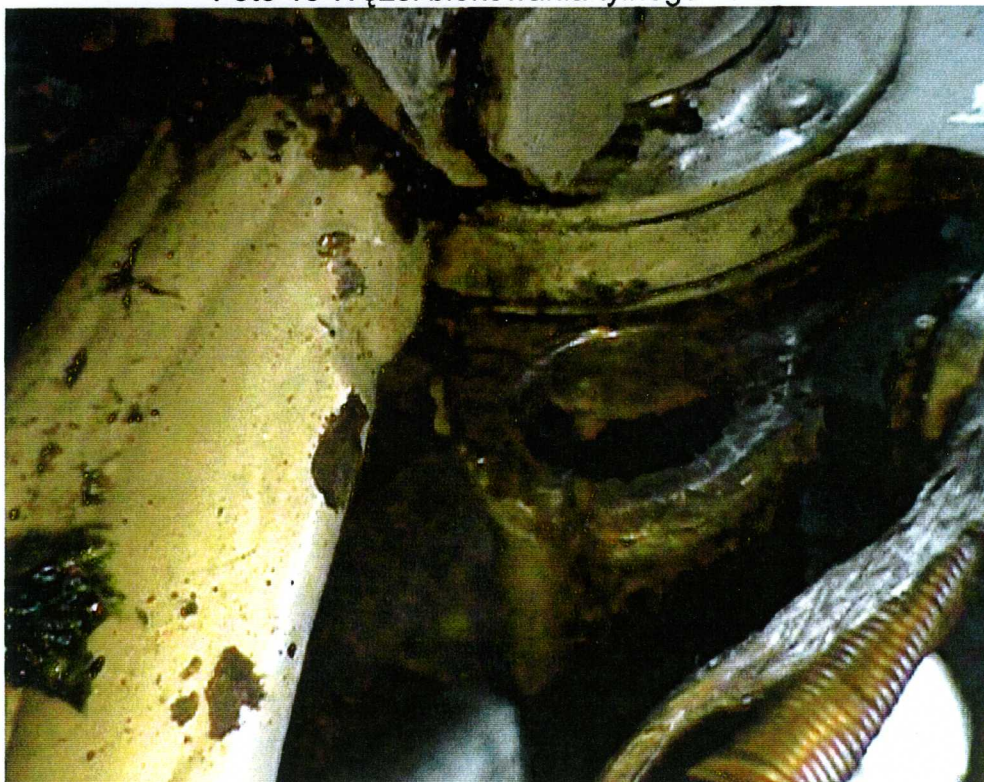
Foto 16 Ucho mechanizmu blokowania kółka tylnego
