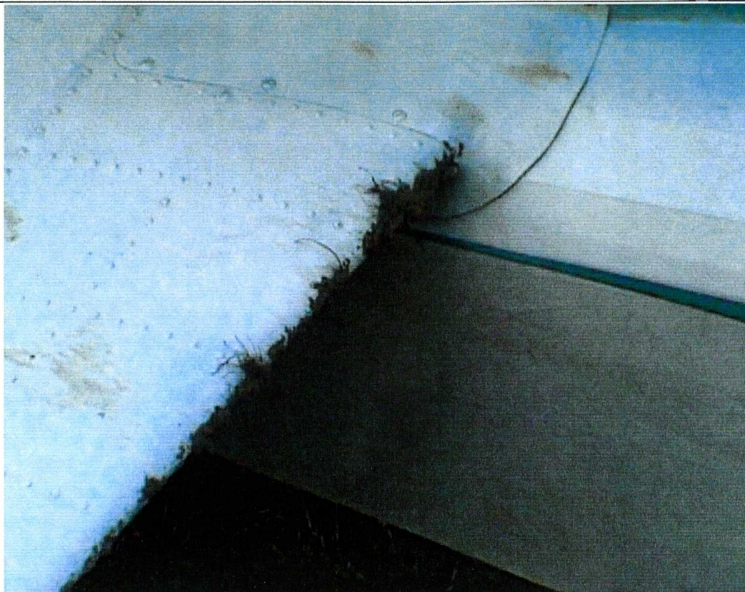
Foto 9 Uszkodzona prawa krawędź natarcia statecznika poziomego
