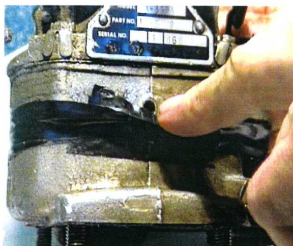
12. Taśma częściowo usunięta – widać otwór bez kulki zaślepiającej.
