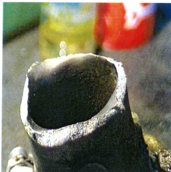
10. Urwany przewód ssący gaźnika.
