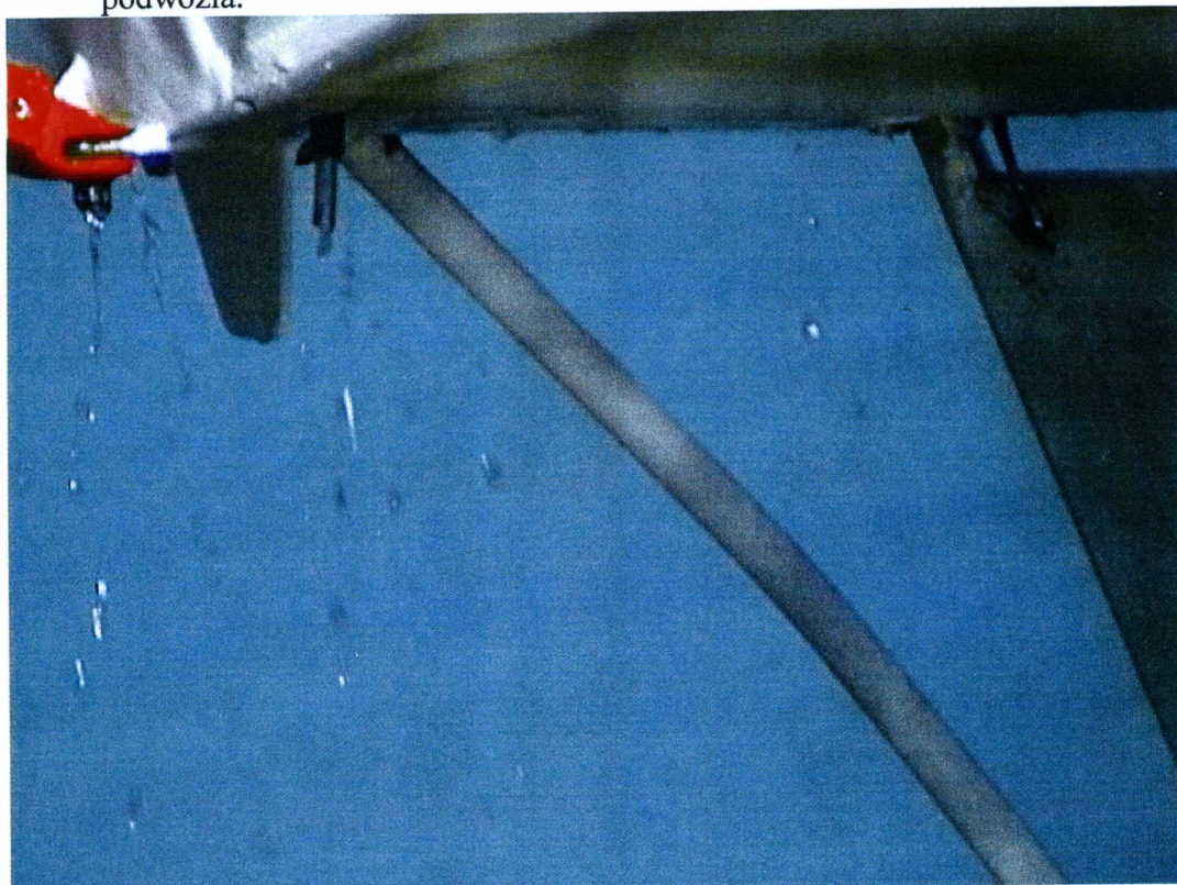
Fot. 6. Wygięcie zastrzału prawego podwozia w powiększeniu.
