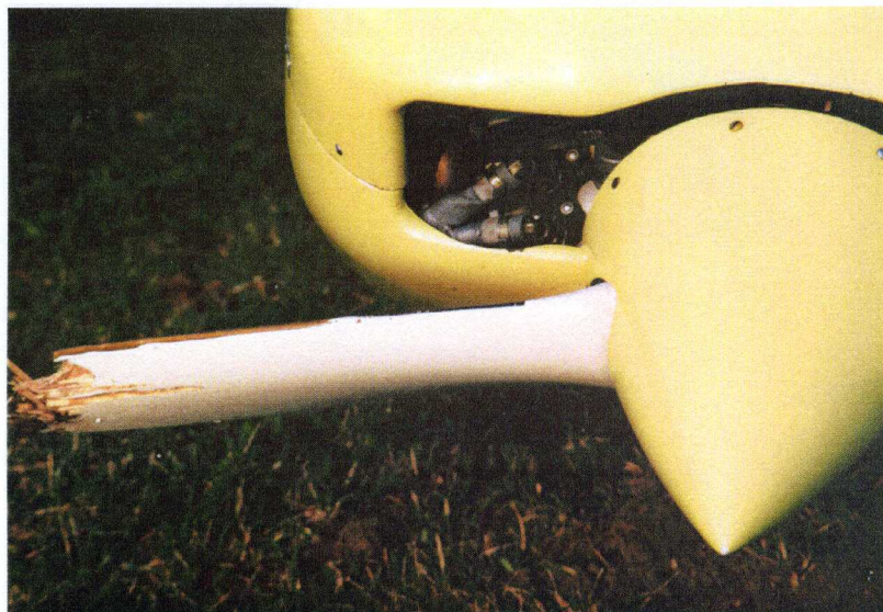
Fot. 4 Widok uszkodzeń jednej łopaty śmigła
