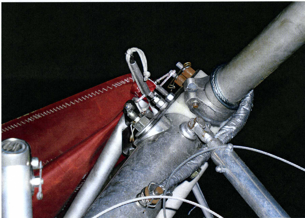
Zbliżenie głównego węzła mocującego
