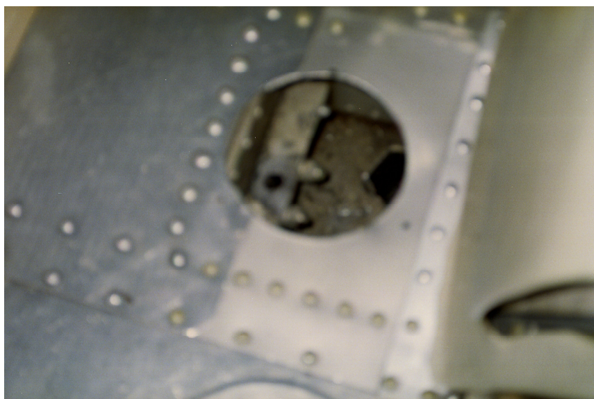
Fot.12 – Wnętrze struktury kadłuba w rejonie uszkodzenia (widok przez wziernik)
