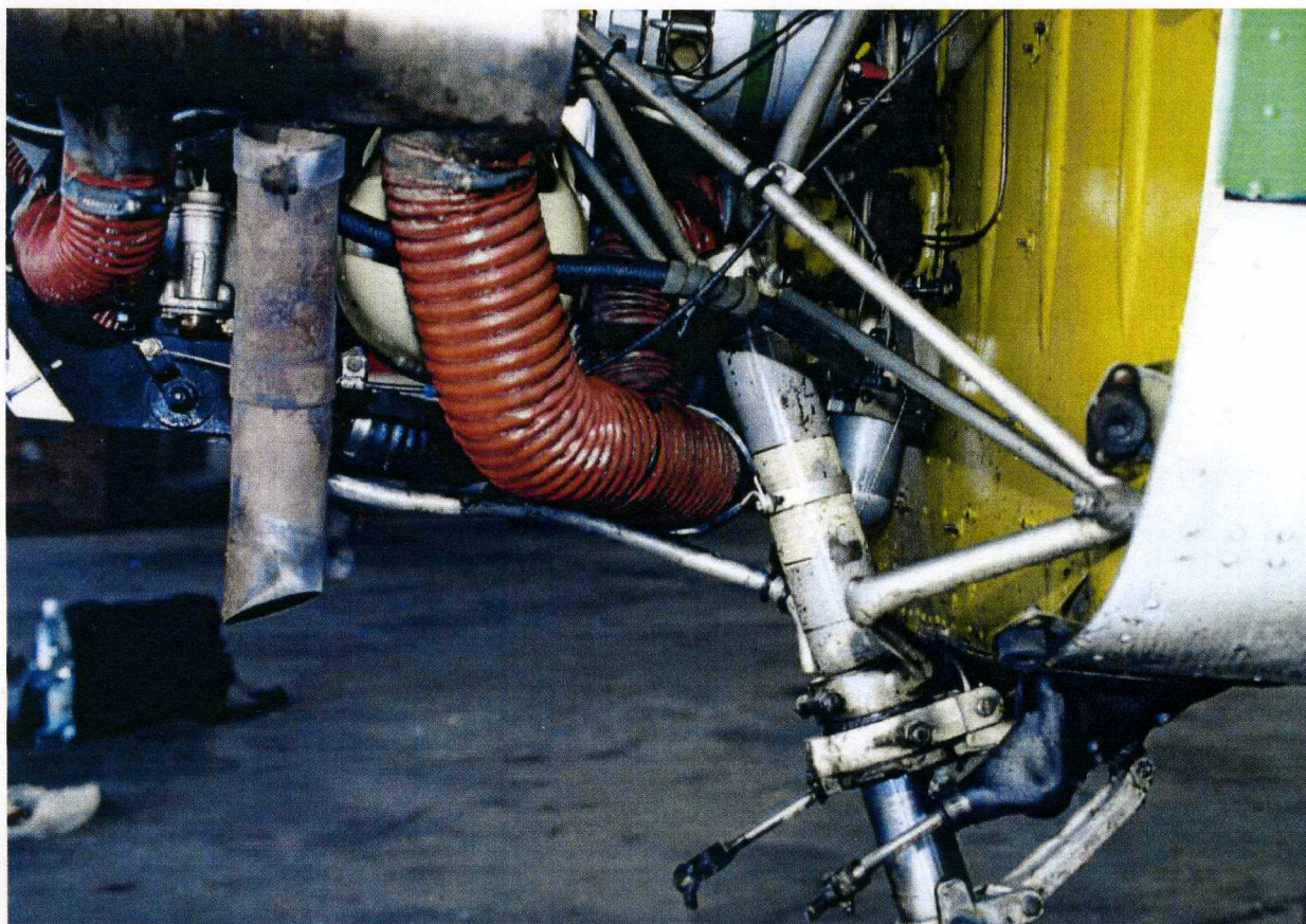
6 – Uszkodzenia podwozia przedniego i łoża silnika.
