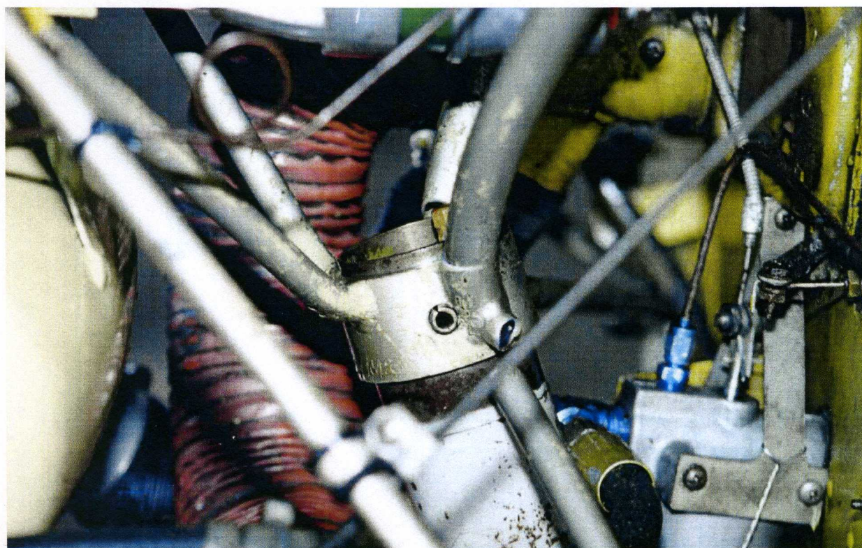
7 – Uszkodzenia podwozia przedniego – górny węzeł mocowania do łoża silnika.
