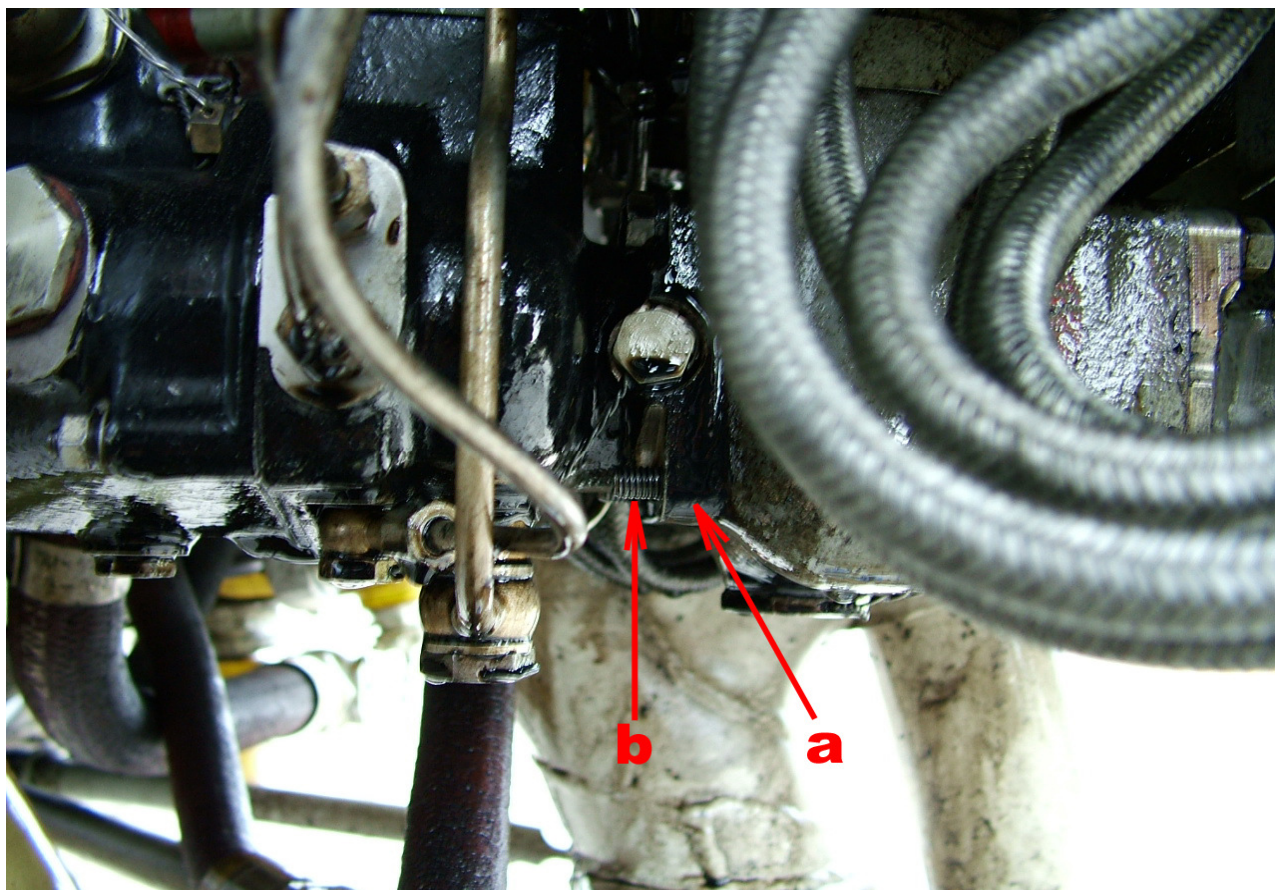
Fot.13 – Widok na silnik z boku w rejonie uszkodzenia: a – kołnierz pompy, b – gwint szpilki bez nakrętki.
