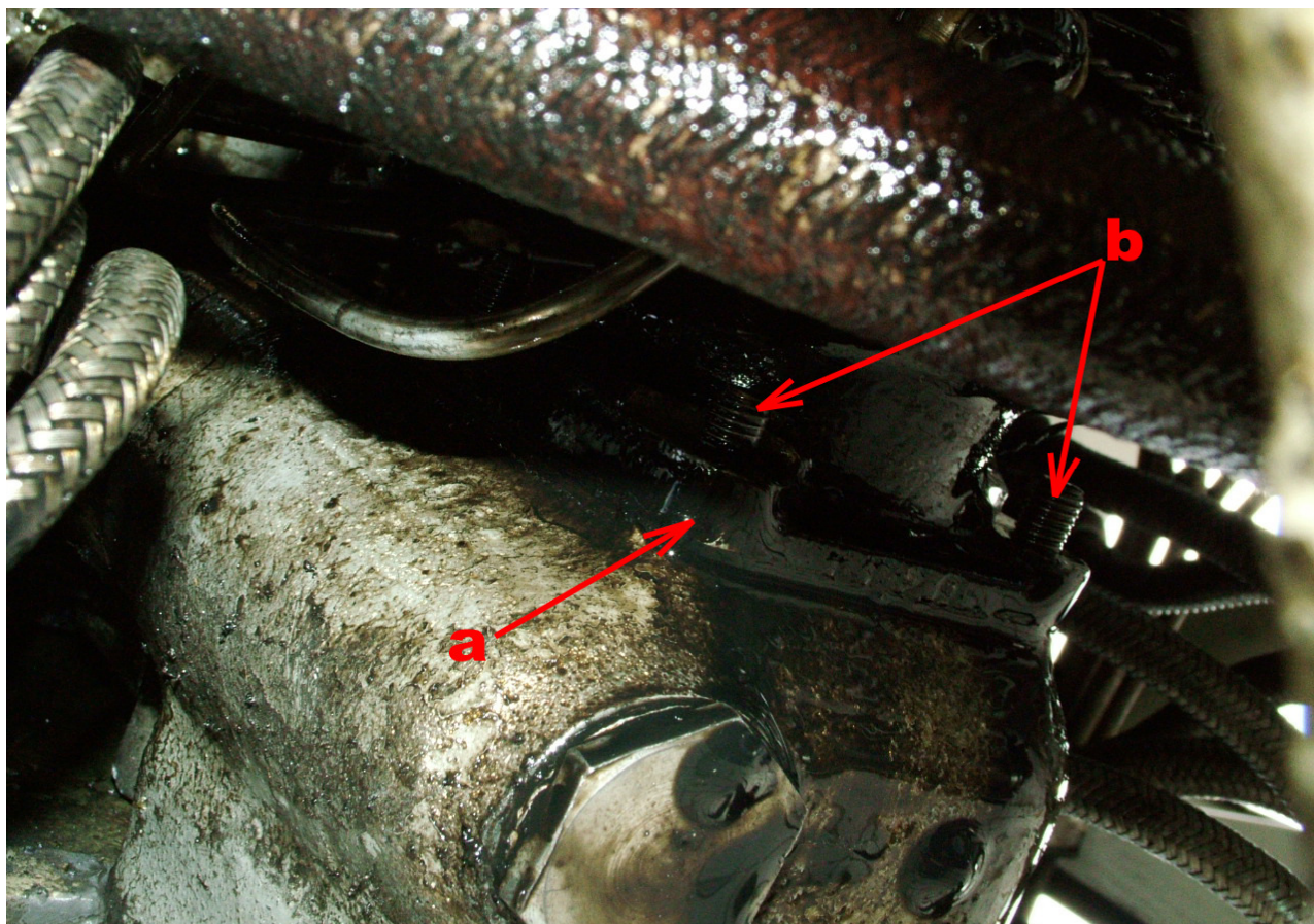
Fot.13 – Widok na silnik z dołu w rejonie uszkodzenia: a – kołnierz pompy, b – gwint szpilki bez nakrętki.
