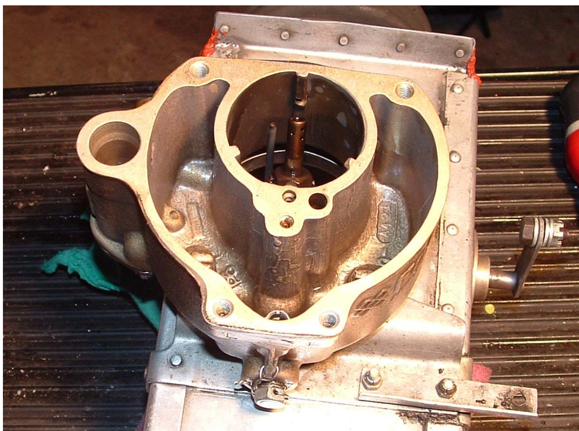
Fot.16 – Rozmontowany gaźnik – komora pływakowa wolna od zanieczyszczeń.
