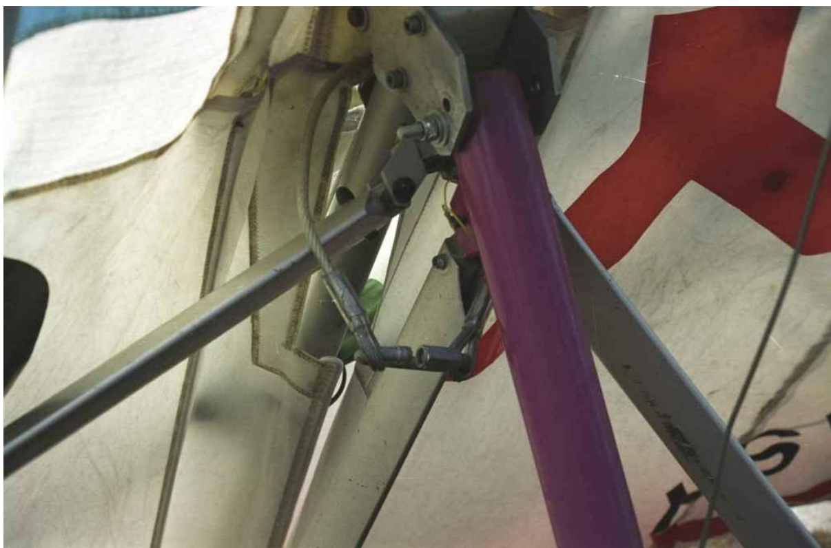
Fot.6 – Główny węzeł skrzydła motolotni z końcówką masztu.
