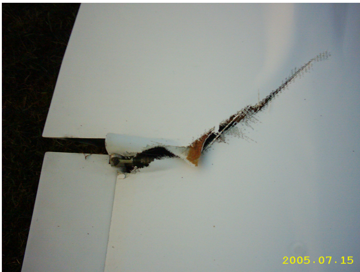
Fot.8 - Uszkodzenia na górnej powierzchni prawego skrzydła w rejonie wyjścia napędu lotki.
