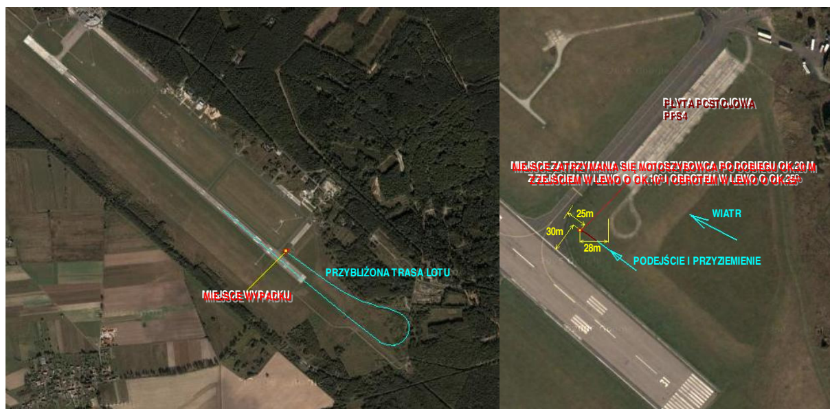
1 – Zdjęcie lotnicze lotniska Szczecin-Goleniów z zaznaczonym miejscem wypadku i szkic sytuacyjny miejsca wypadku.
