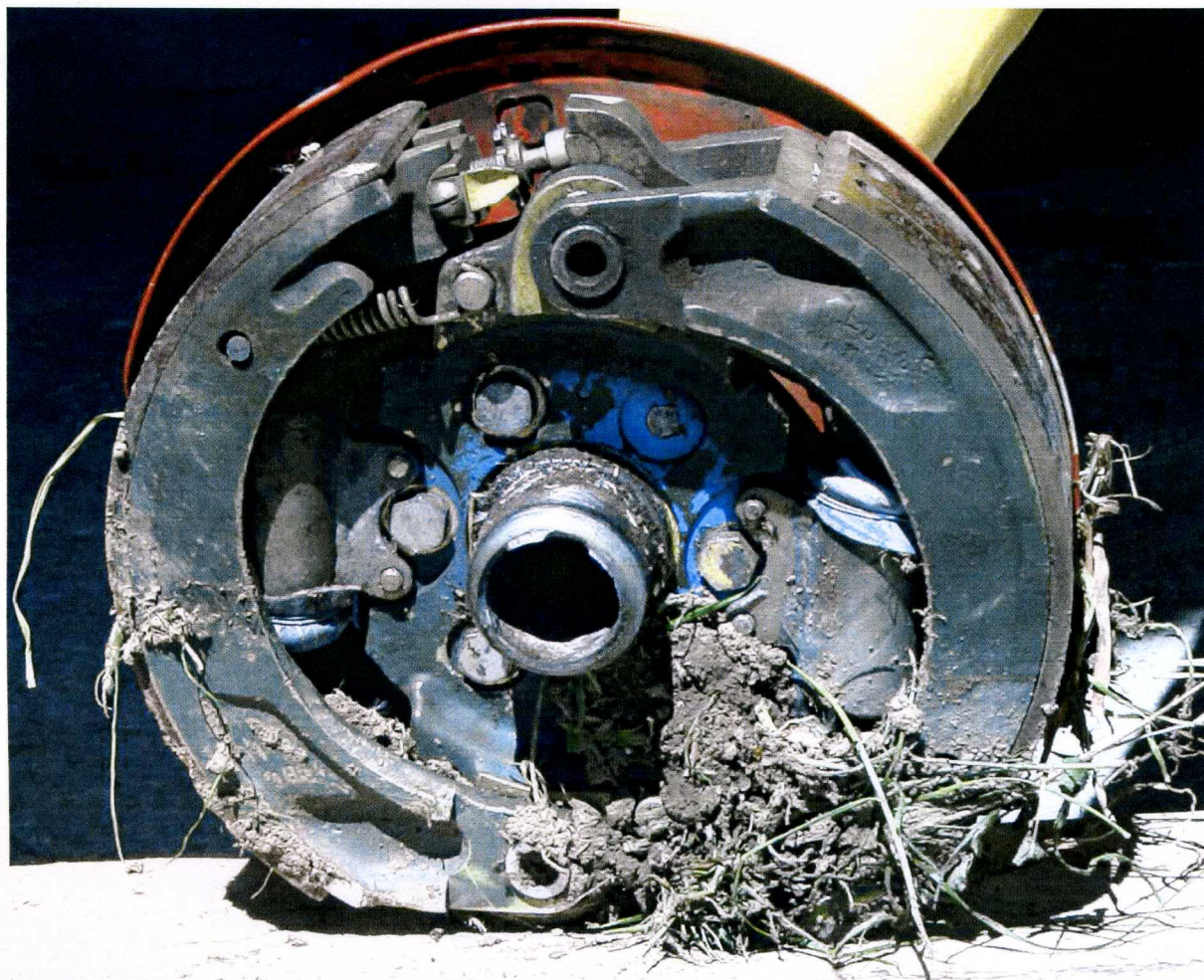
Fot.15 – Widok uszkodzonego zespołu bębna hamulcowego i osi.
