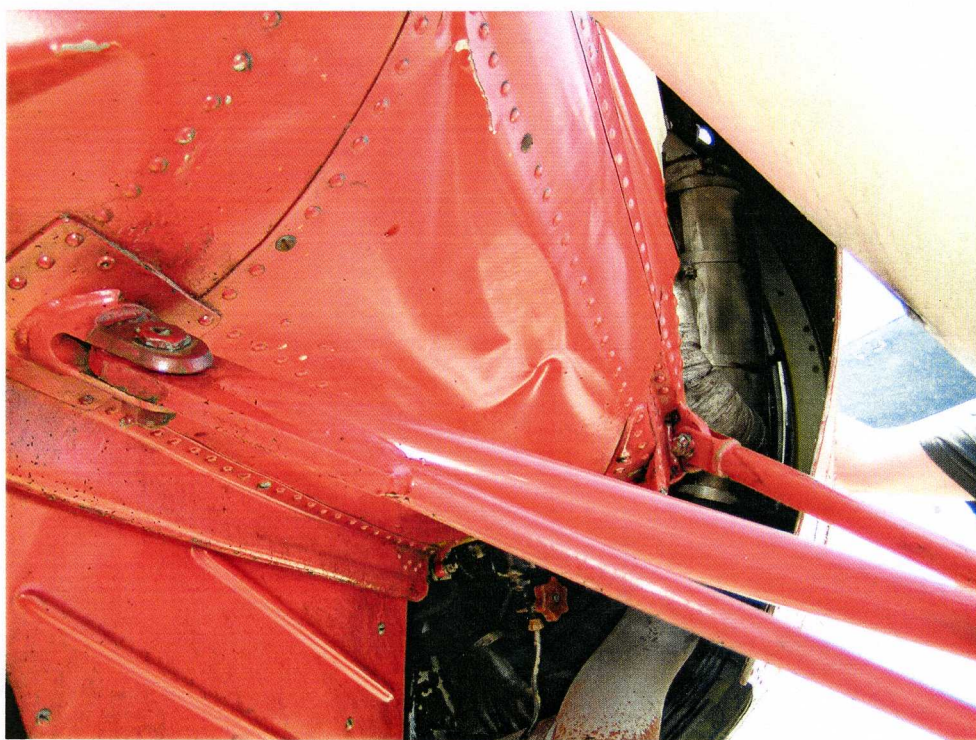
Fot. 8 – uszkodzenie blach dolnego pokrycia kadłuba za silnikiem – strona prawa
