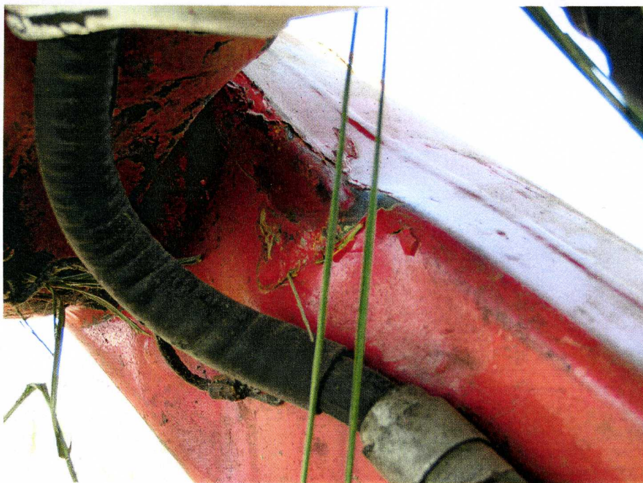
Fot. 2 – uszkodzenie prawego wahacza podwozia głównego
