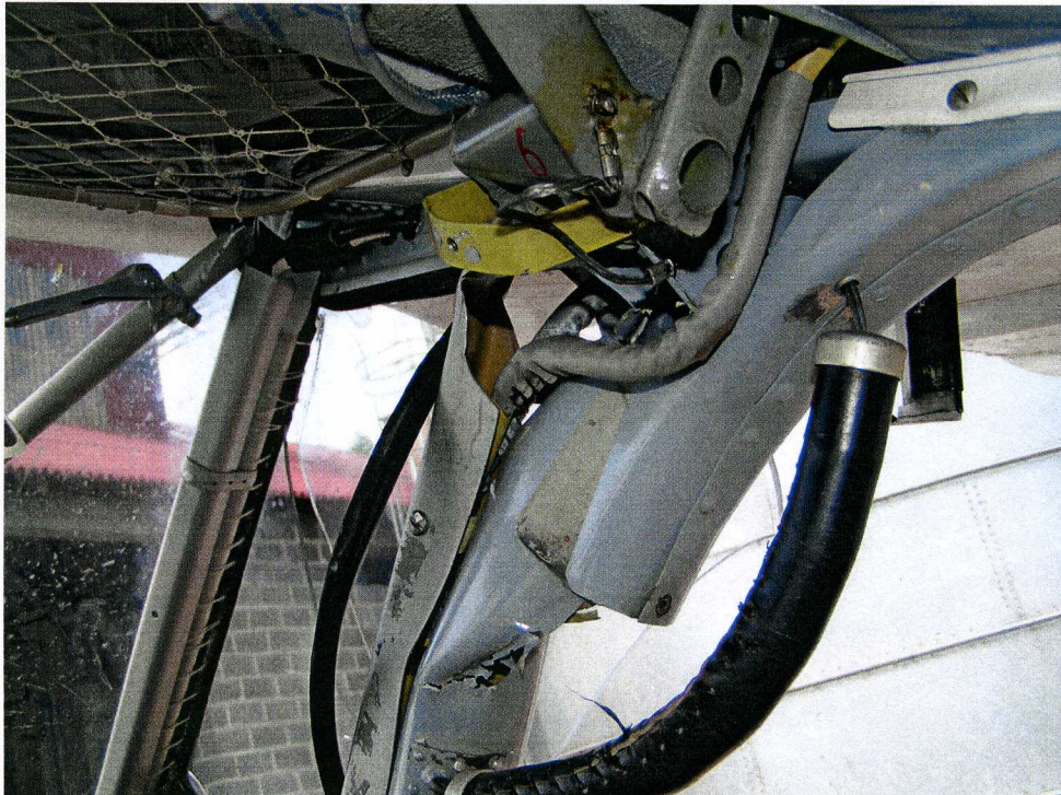
Fot. 4 – uszkodzenie wręgi nr 2 - szczegół
