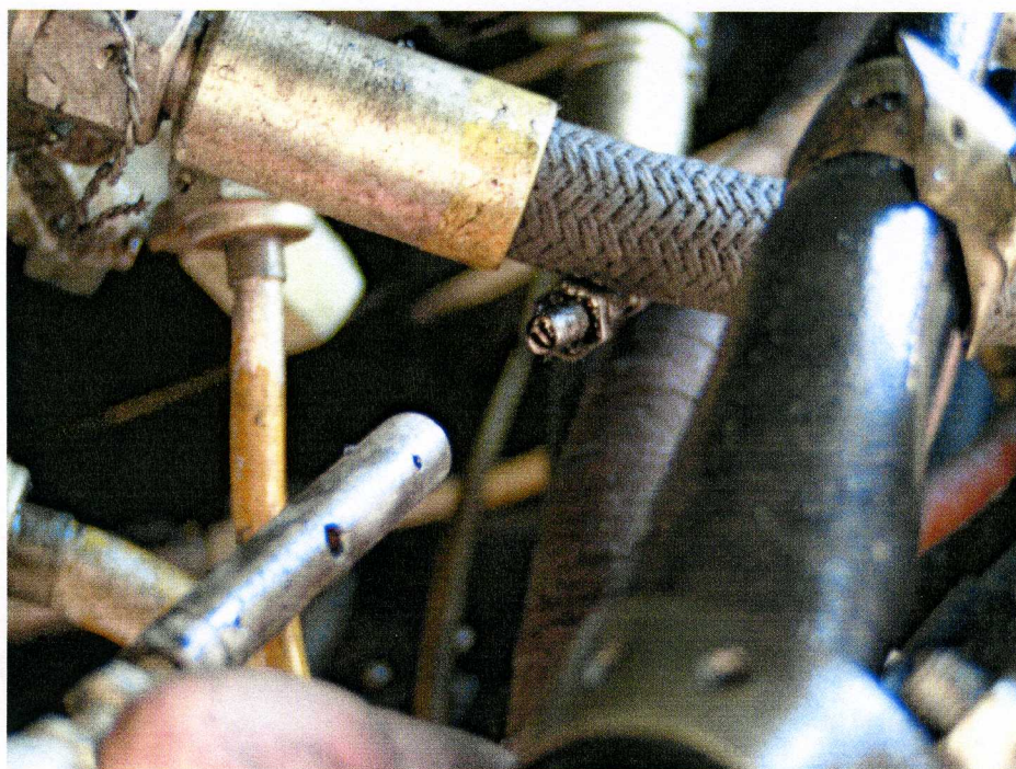
Fot. 1 – rozłączone cięgno sterowania poprawki wysokości
