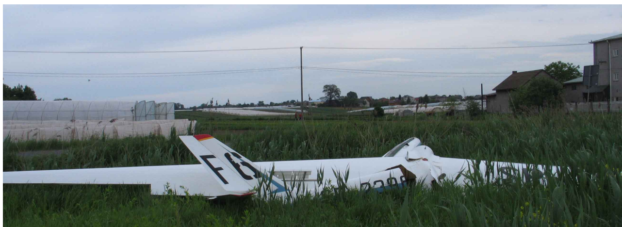
4 – Widok rozbitego szybowca w kierunku przeciwnym do kierunku podejścia.
