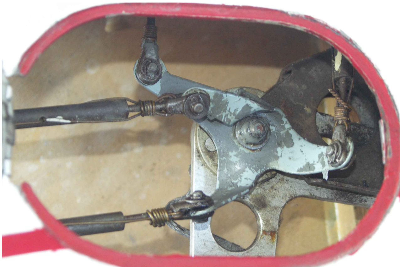
23 – Zbliżenie otwartego wziernika – dobrze widoczne dźwignie sterowania sterem wysokości i ich uszkodzenia.
