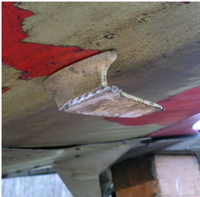
Fot.13 – Uszkodzenia spodu kadłuba, widoczna złamana antena.
