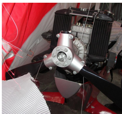
17 i 18 – Zespół napędowy pokazany z tyłu i z prawej strony od dołu, widoczne śmigło z odłamaną łopata
