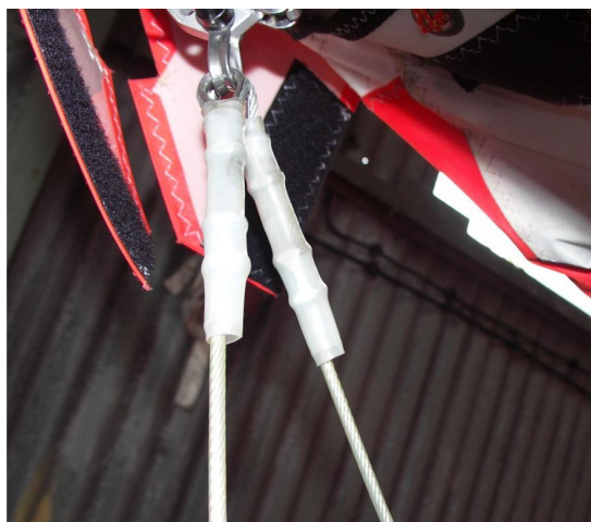
5 – Nosek kila z linkami.
