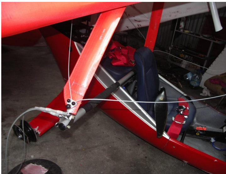
10 – Prawa strona wózka, widoczne mocowanie linek do prawej strony trójkąta i uszkodzone podwozie główne.
