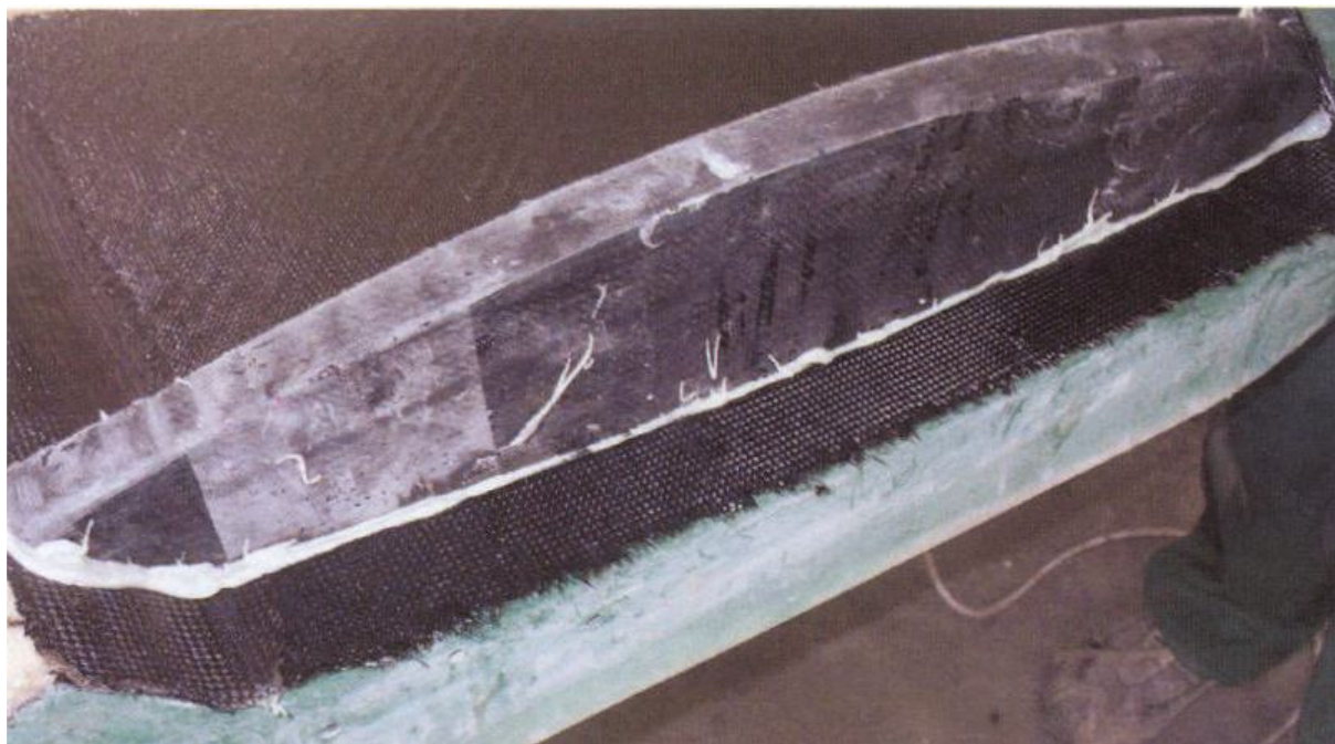
6 – Nasadowe żebro lewego skrzydła w trakcie klejenia do dolnego pokrycia, jeszcze bez wykonanych otworów odpowietrzających wewnątrz struktury.
