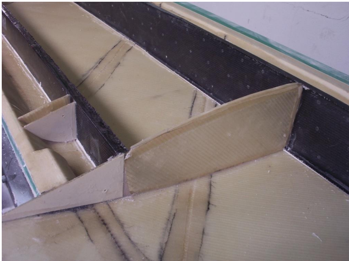
5 – Wnętrze struktury skrzydła (bez górnego pokrycia) w rejonie rozklejenia.
