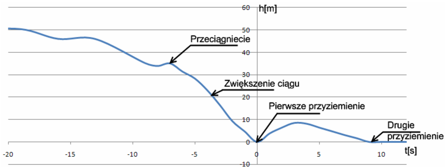
4. – Wykres wysokości lotu w funkcji czasu. Czas t=0 w pierwszym punkcie przyziemienia (czas 0:21 na zdjęciach 3.).
