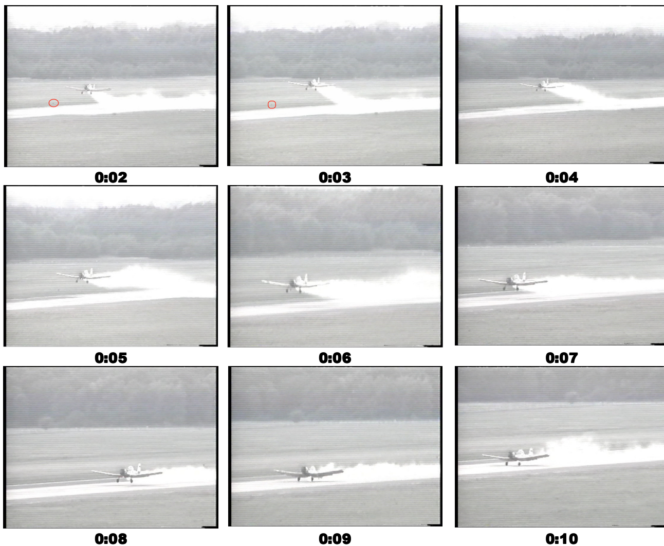
3cd. – Zapis z kamery wideo rejestrujący wypadek.
