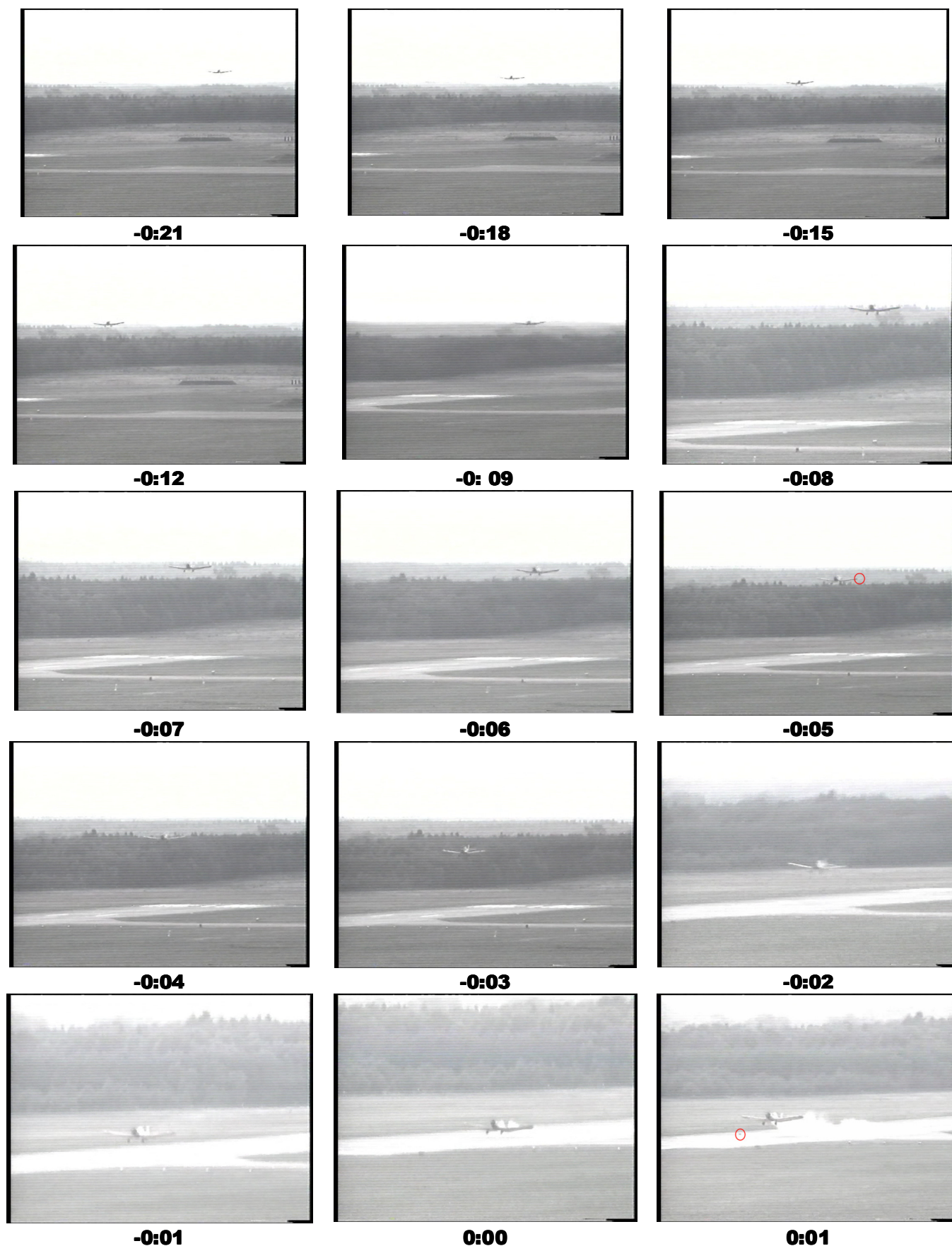
3. – Zapis z kamery wideo rejestrujący wypadek. Na zdjęciu -0:05 czerwonym kolorem zaznaczono wir powstały na końcówce skrzydła w skutek przeciągnięcia. Na zdjęciu 0:01 czerwonym kolorem oznaczono tylne koło oderwane od samolotu.
