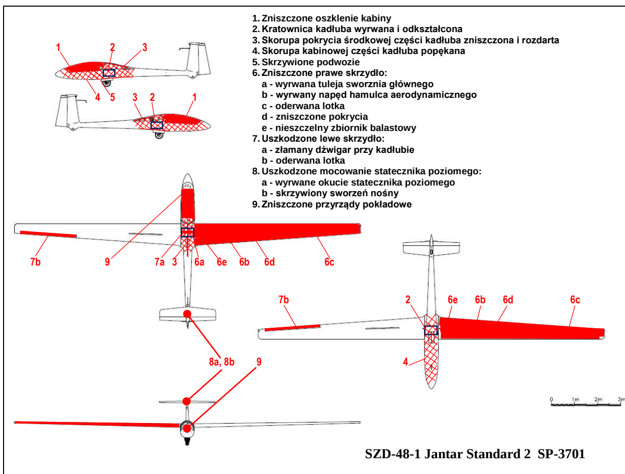
4 – Stan szybowca po wypadku – uszkodzenia i zniszczenia naniesione schematycznie na jego rysunki w rzutach.
